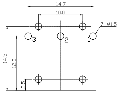
PCB板安装孔图
